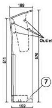
right 右側
